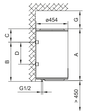
INSTALACIÓN VERTICAL
